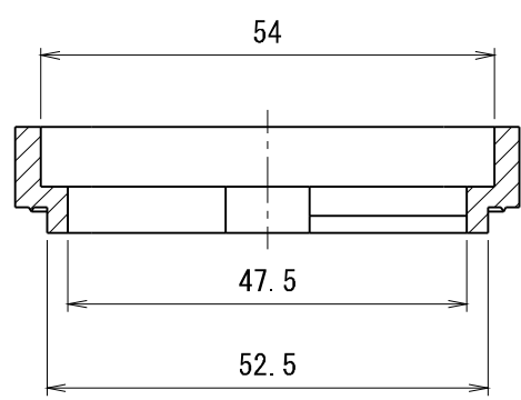
断面 A-A
